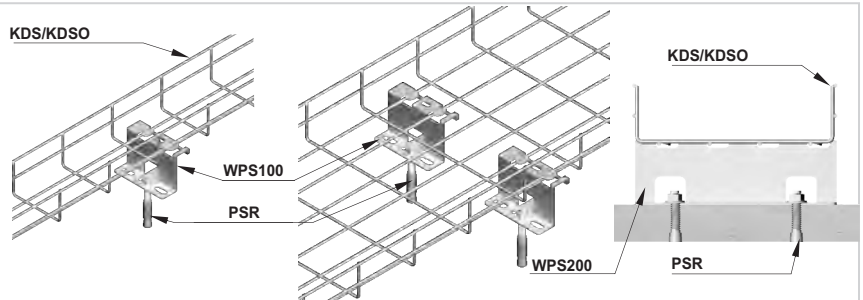
Пример использования напольного кронштейна WPS100 и WPS200.
