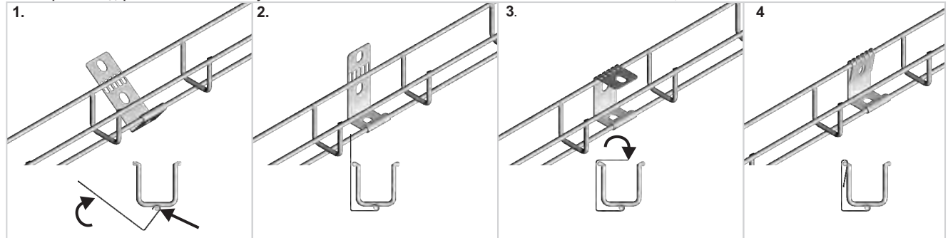
Пример использования держателя USKM35 с кронштейном WW
