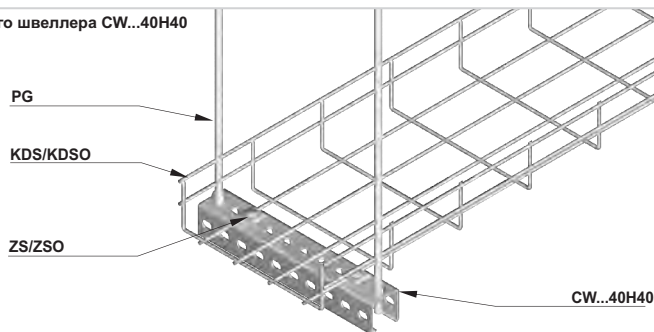
Пример использования усиленного швеллера CW...40H40
