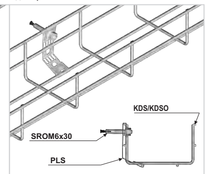
Пример использования полосы PLS для крепления к стене
