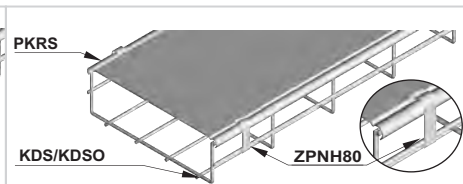
Пример использования защелки ZPNH80
