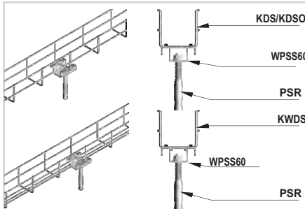
Примеры использования настенно-напольного кронштейна WPSS - крепление к стене
